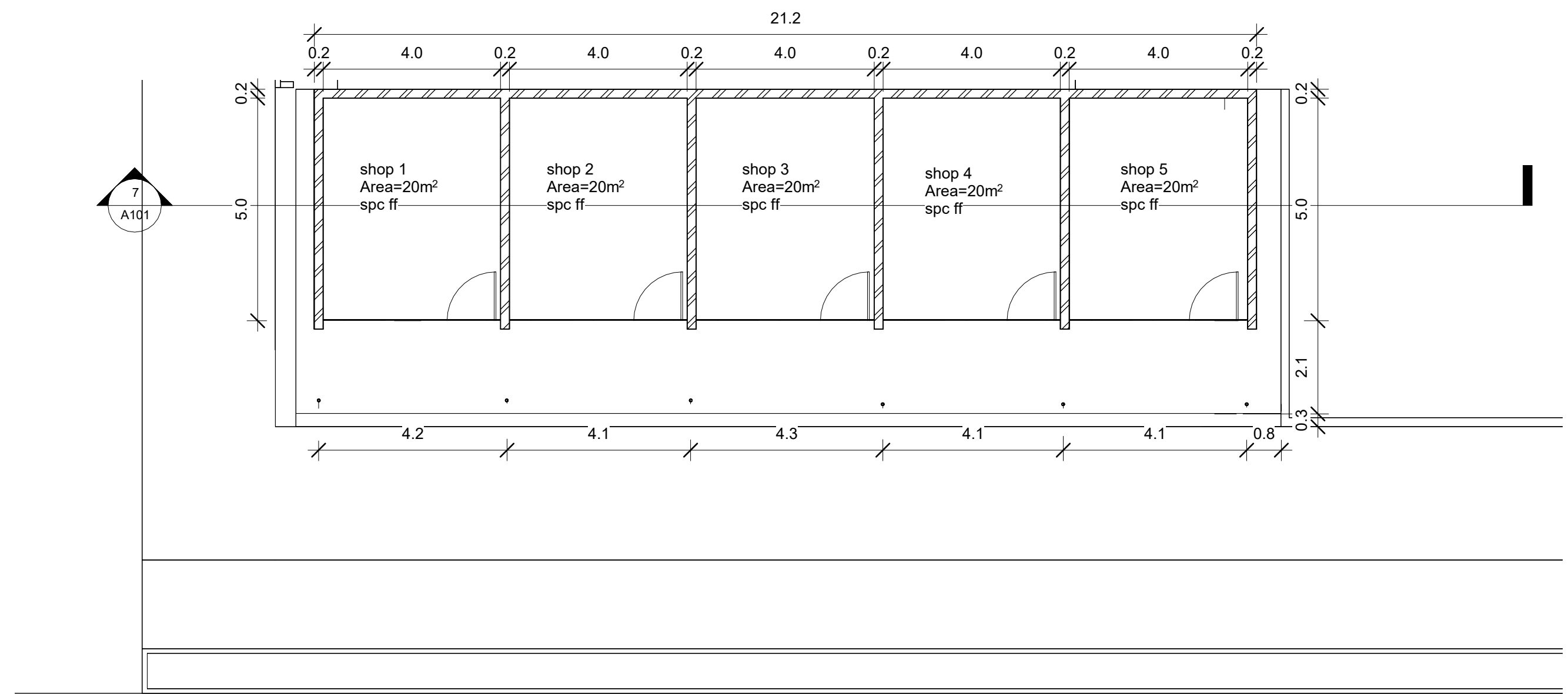
6 FLOOR PLAN 1 : 100
