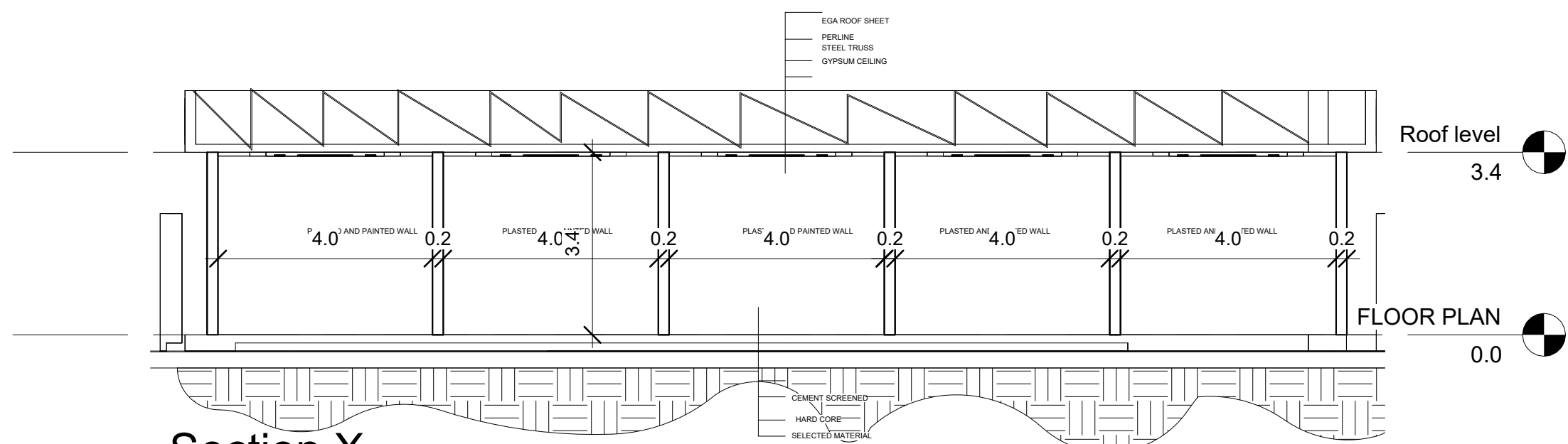
7 Section X 1 : 100
