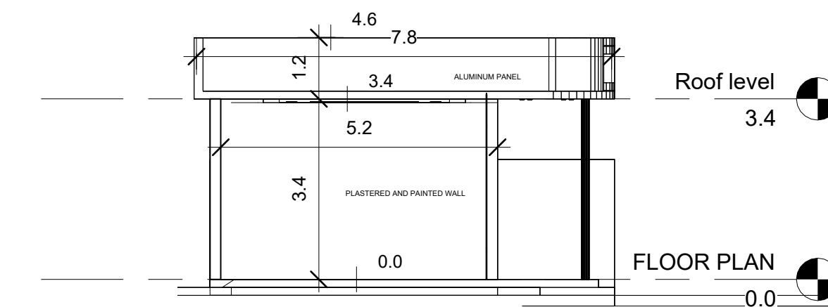
1 RIGHT ELEVATION 1 : 100
